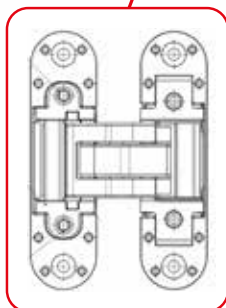
3D Regelbare verdoken scharnieren / Charnières masquées réglables 3D
