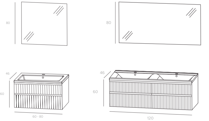
Set incl. glanzend witte keramische wastafel + spiegel. Set avec plan céramique blanc brillant + miroir.
