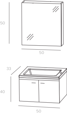
Set incl. glanzend witte polybeton wastafel + spiegelkast. Set avec plan polybéton blanc brillant + AMT.
