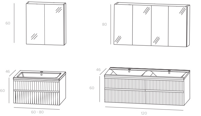
Set incl. glanzend witte keramische wastafel + spiegelkast. Set avec plan céramique blanc brillant + AMT.
