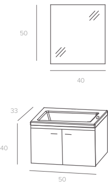
Set incl. glanzend witte polybeton wastafel + spiegel. Set avec plan polybéton blanc brillant + miroir.
