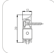
Opbouw valdorpel Kaltefein à poser
